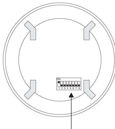
Μικροδιακόπτες επιλογής διεύθυνσης στην κάτω πλευρά του ανιχνευτή
