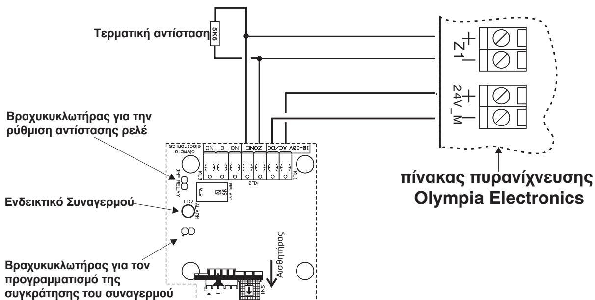
Σχήμα 2. Σχεδιάγραμμα σύνδεσης με πίνακα πυρανίχνευσης Olympia Electronics.
