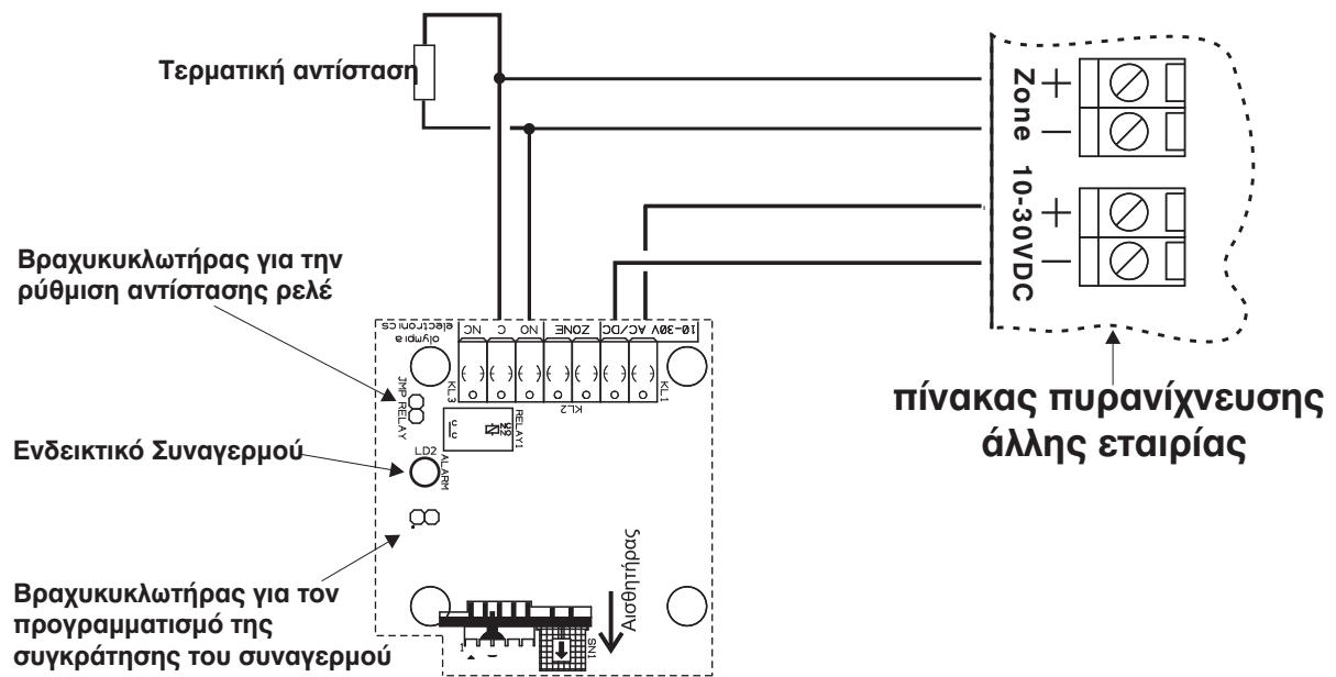
Σχήμα 3. Σχεδιάγραμμα σύνδεσης με πίνακα πυρανίχνευσης άλλης εταιρίας.
